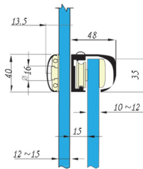
Instalación a Vidrio
